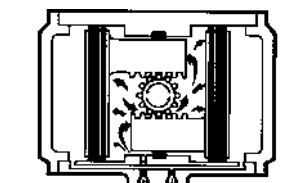
“A”口进气驱动轴反时针旋转
