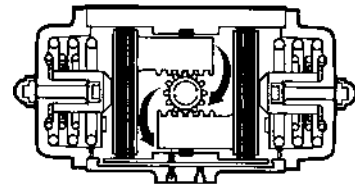
“B”口排气驱动轴正时针旋转
