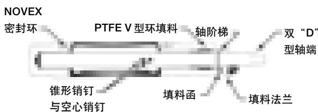
典型阀门结构
